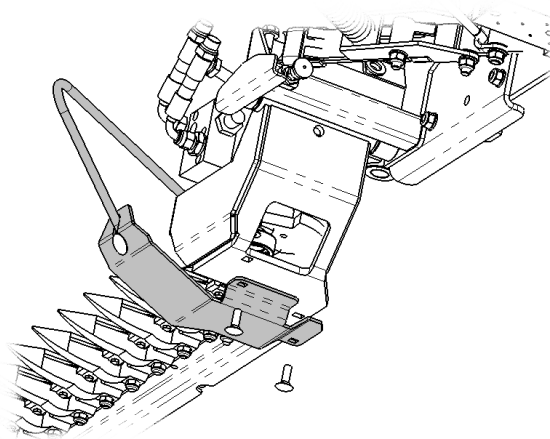
Klippsats för högt gräs, undersidan av balken
