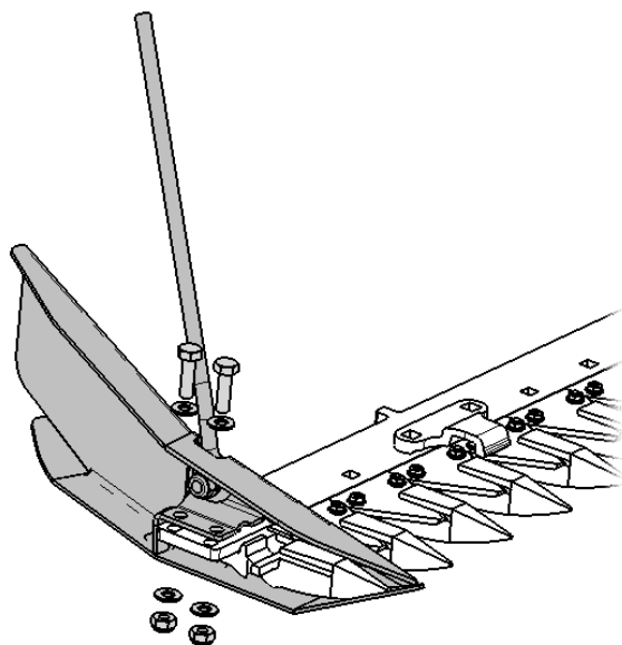
Klippsats för högt gräs, änden på balken
